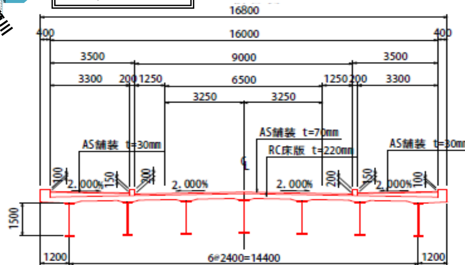
上部工断面図
