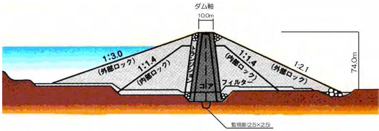
図 19 網木川ダム堤体断面図
