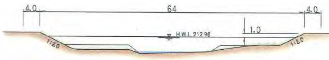
図 15 屋代川代表横断図（吉野川合流点から上流 0.3km、単位：m）
