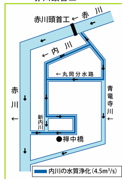
&lt;内川浄化用水導水ルート&gt;
