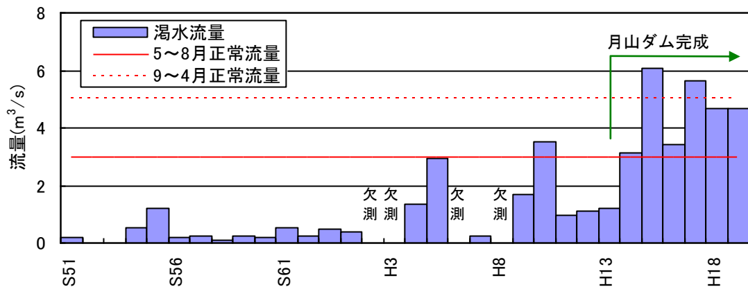
<渇水流量の経年変化(熊出地点)>
