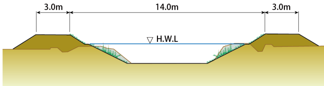
<矢引川 整備イメージ>
