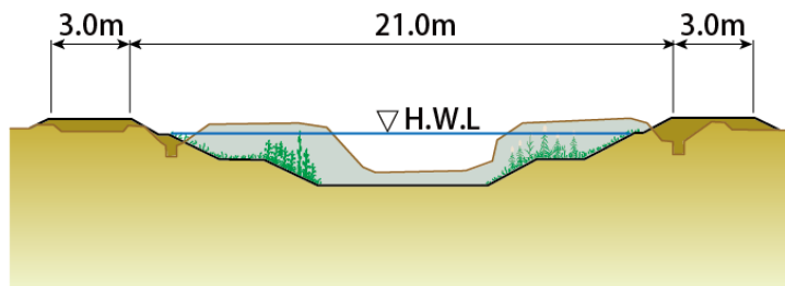
<湯尻川 整備イメージ>
