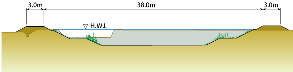
目標流量75m 3 /s区間の標準断面図
