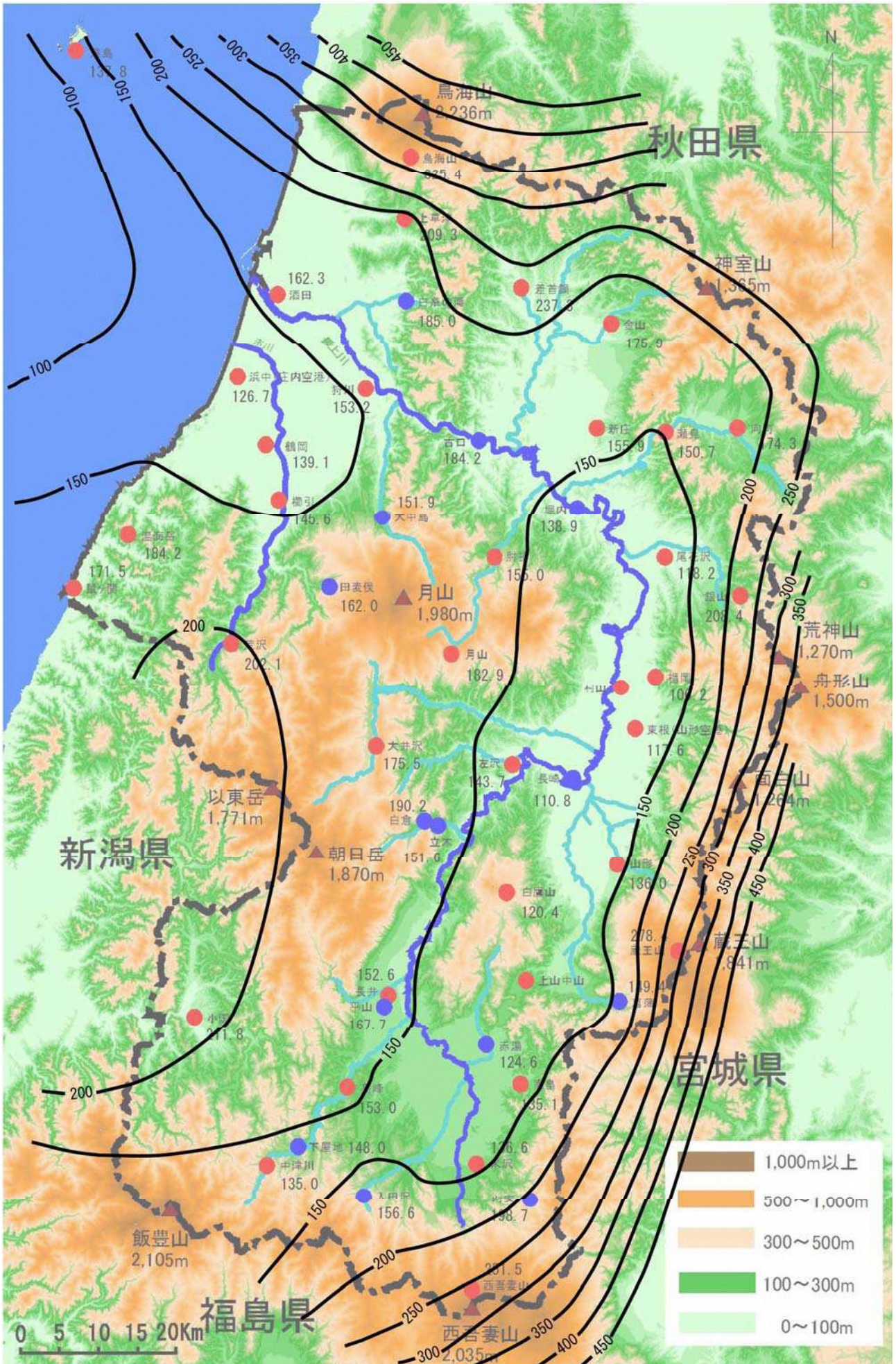
30年確率日雨量等雨量線図
