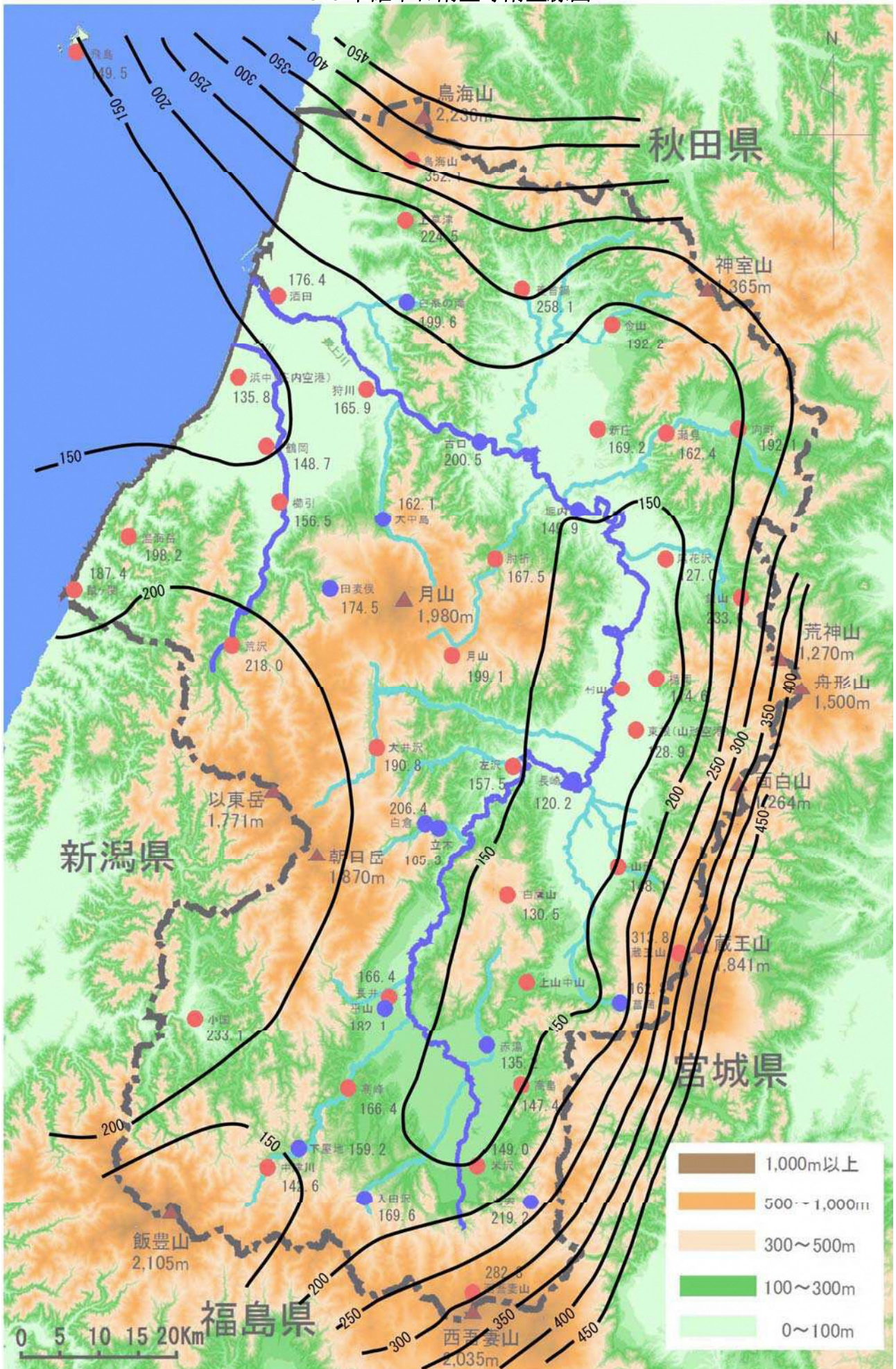
50年確率日雨量等雨量線図
