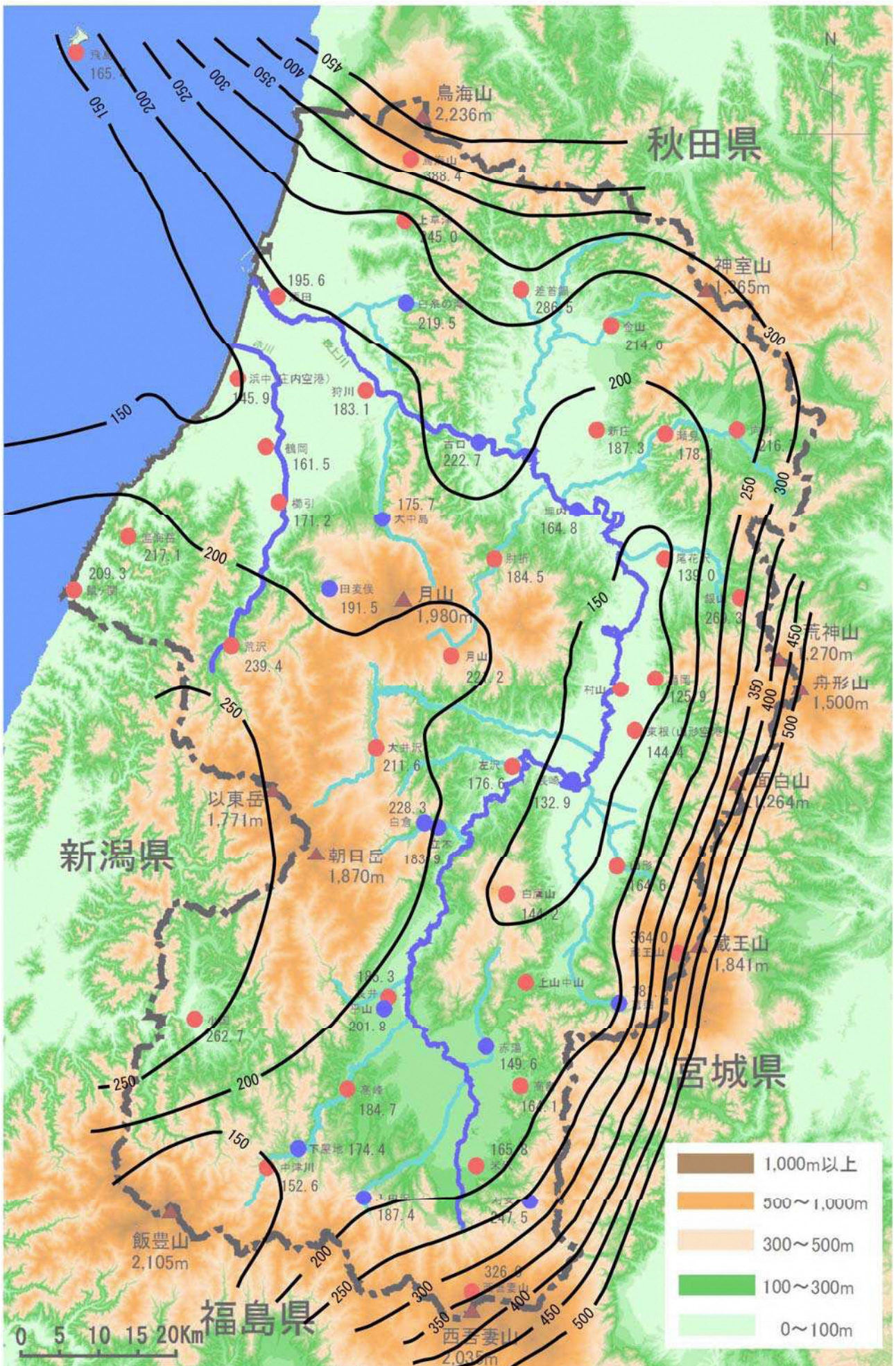
100年確率日雨量等雨量線図
