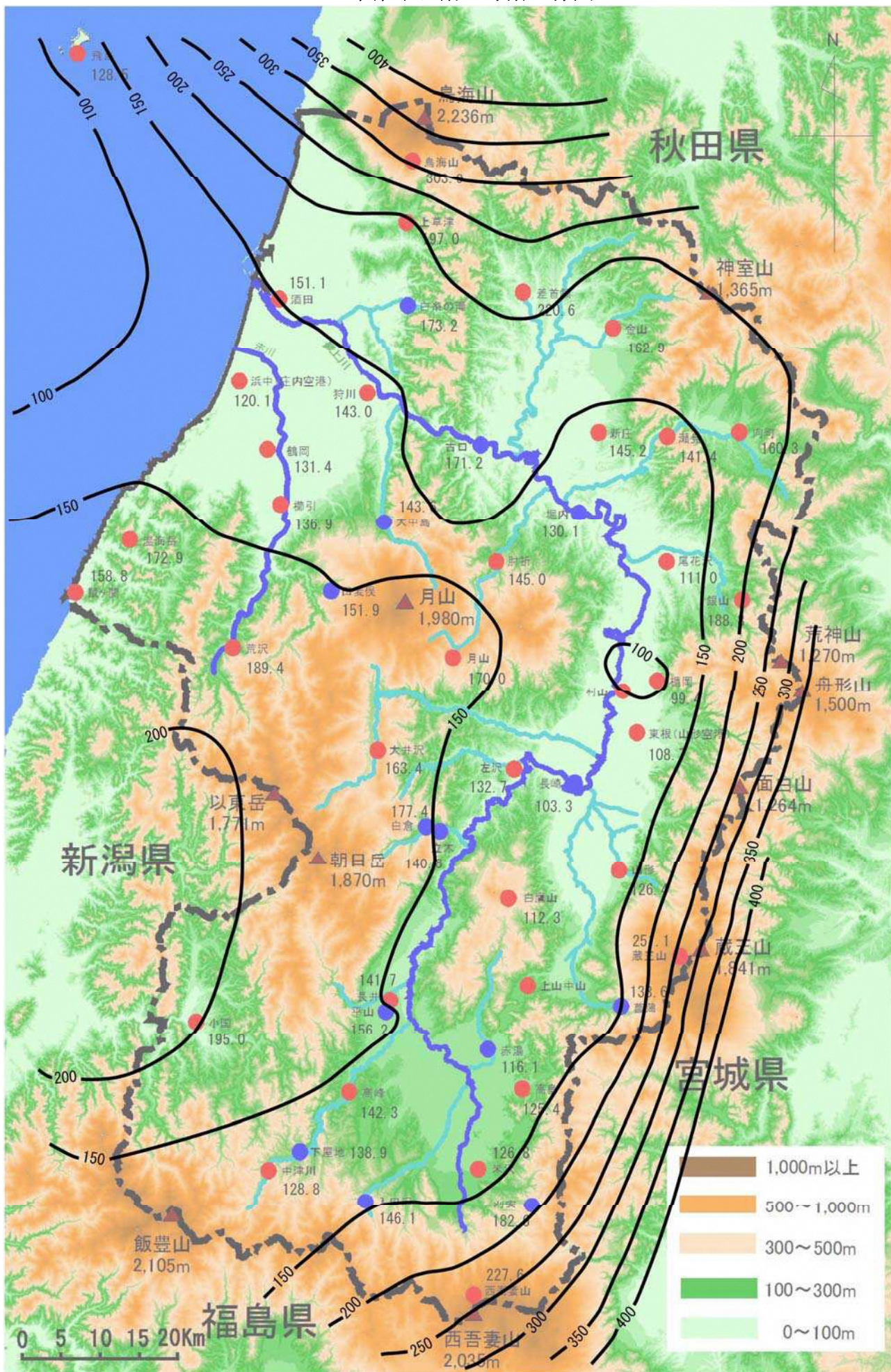
20年確率日雨量等雨量線図
