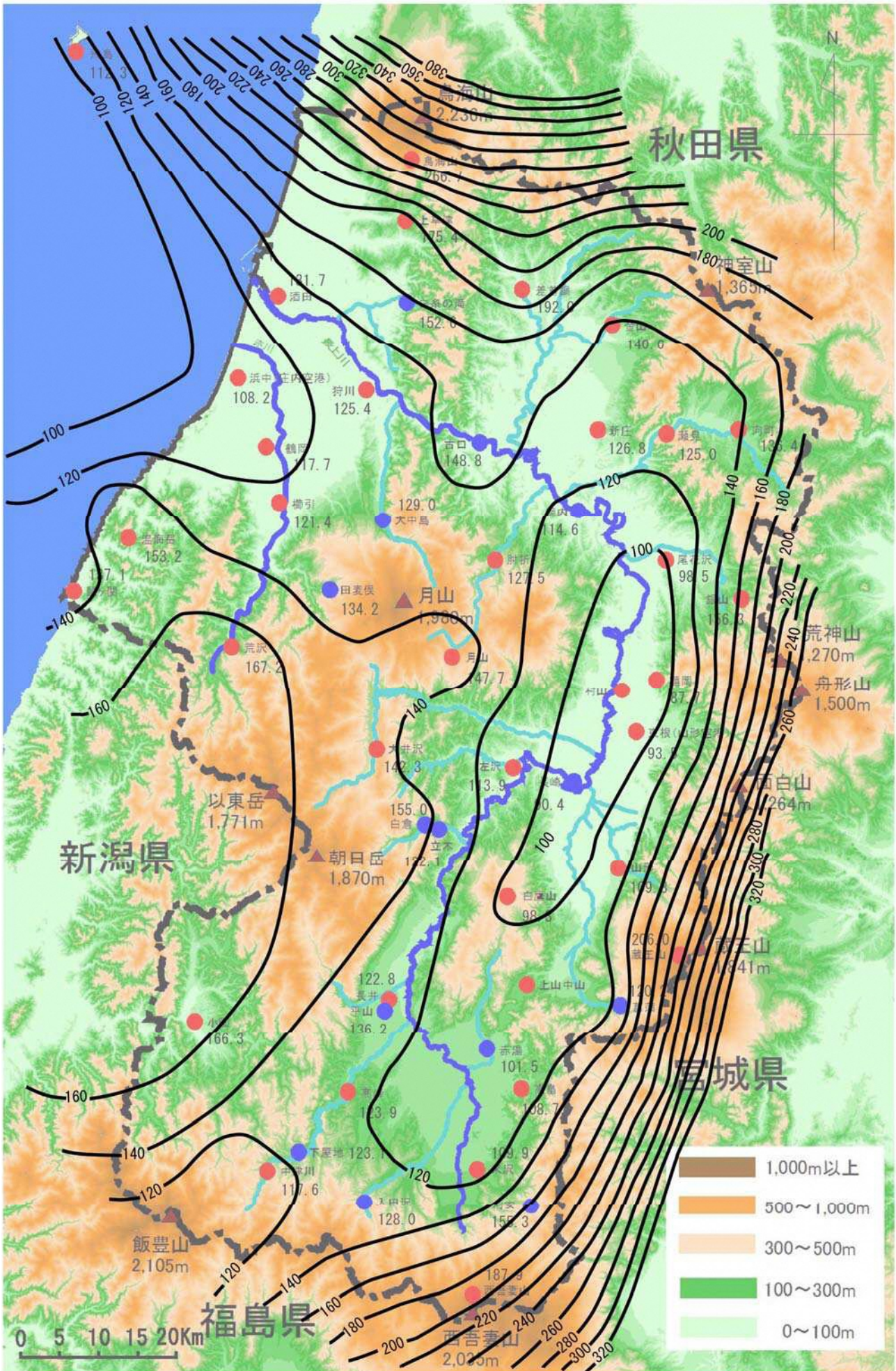
10年確率日雨量等雨量線図
