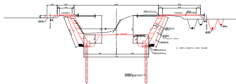
計画断面図
