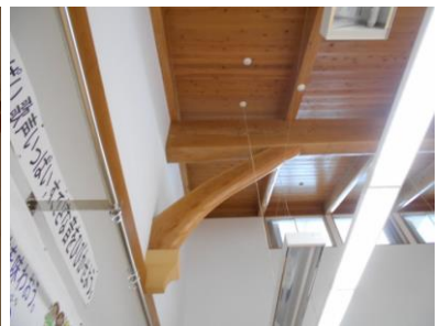
下写真: 特徴ある建築デザイン、根曲り材を法杖や筋交的に利用、太鼓落し材が多い
