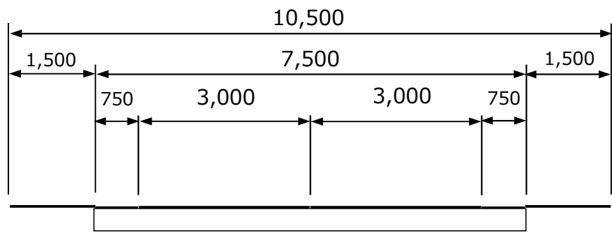
現況横断図
