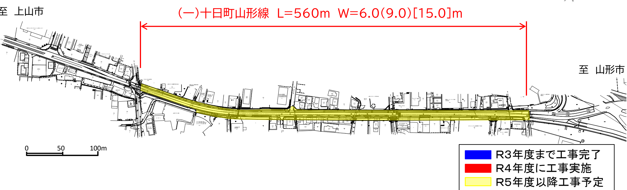
計画平面図
