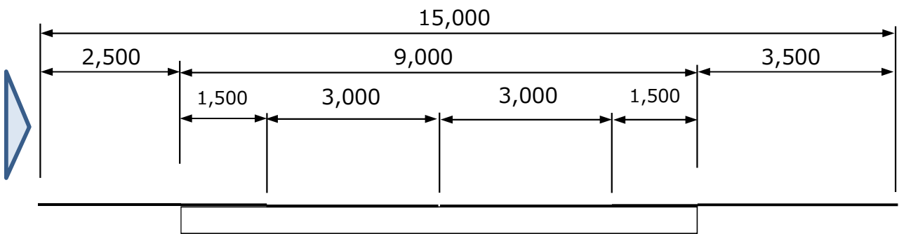
計画横断図
