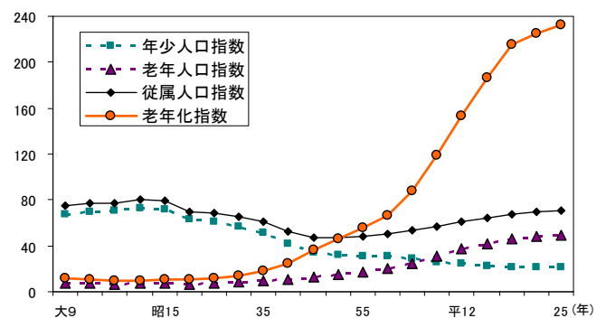
図8 年齢構造指数の推移(大正9年～平成25年)
